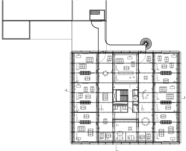
3. Obergeschoss
