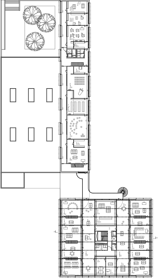
2. Obergeschoss
