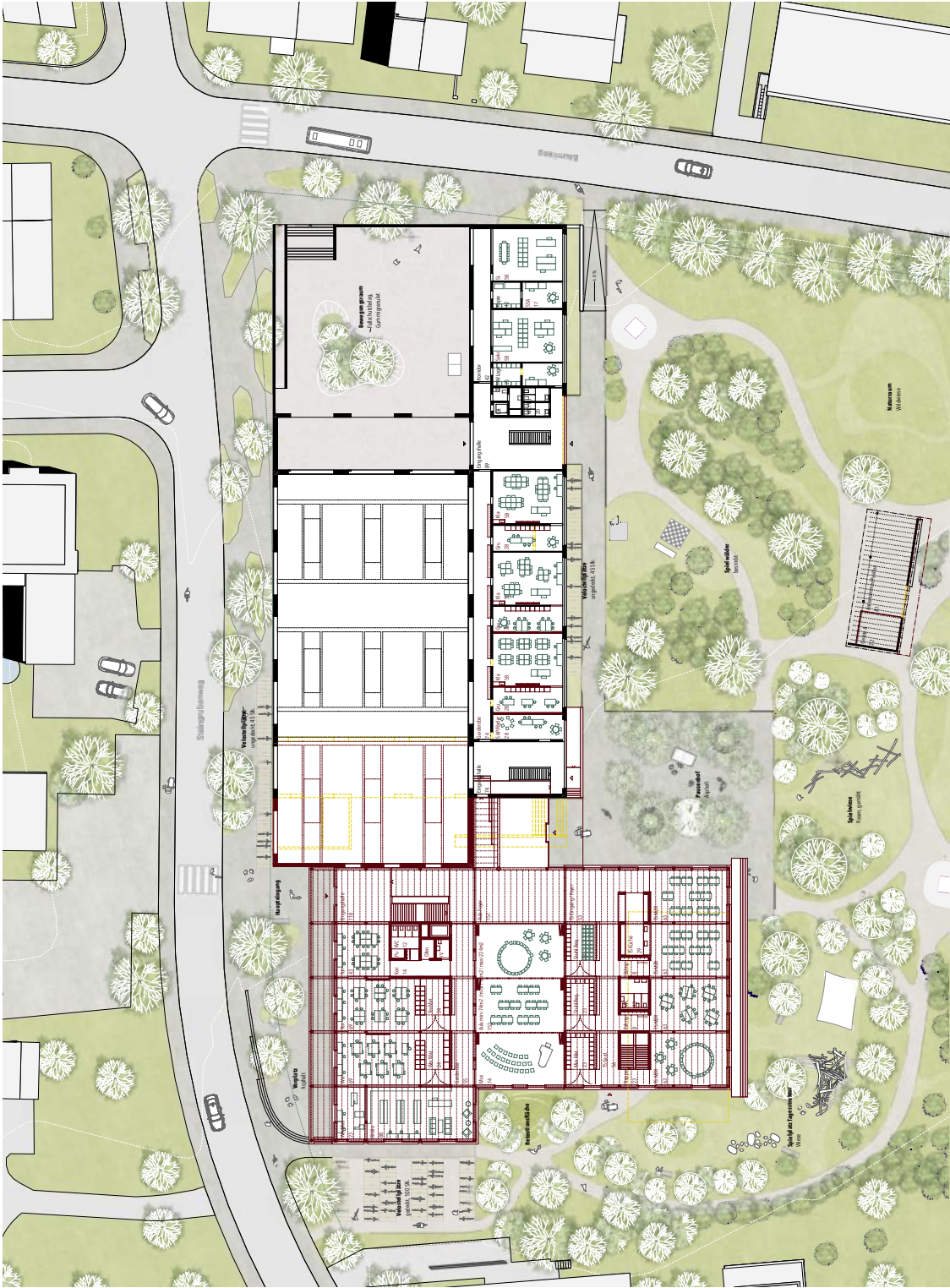
Erdschloß Anbindung Umgebung M 1:200
