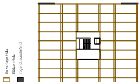
Tragwerk Konzept 1:300
