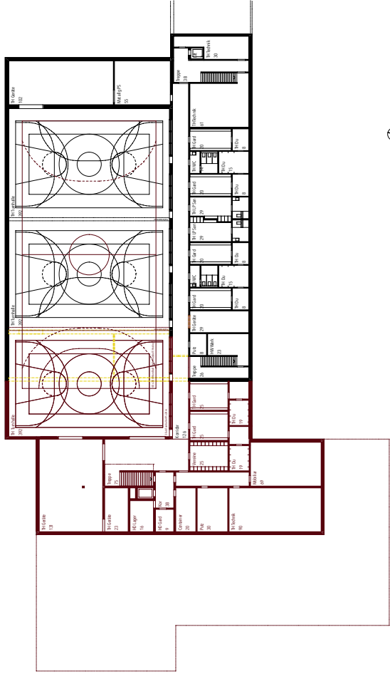
Untergeschoss
